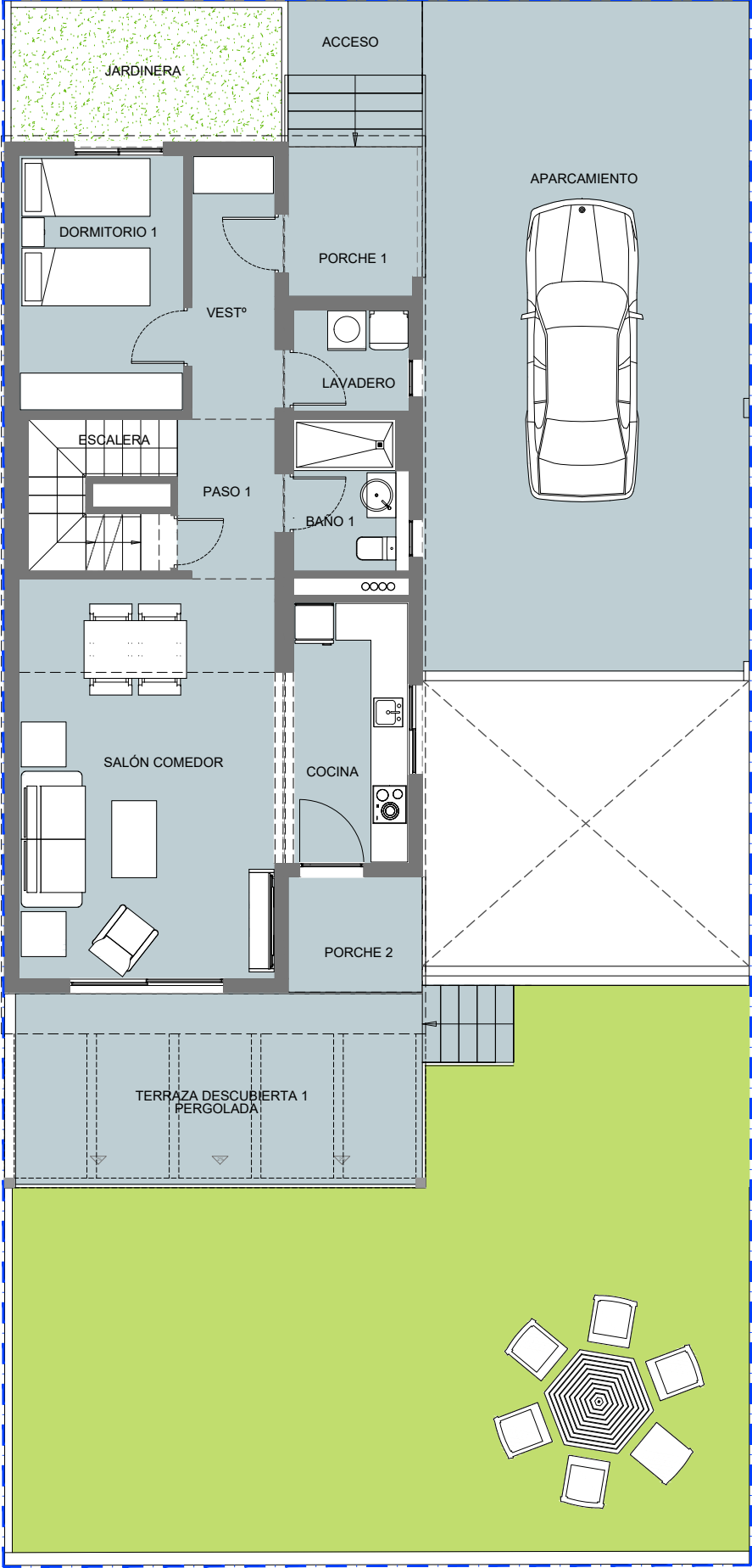
PLANTA BAJA
