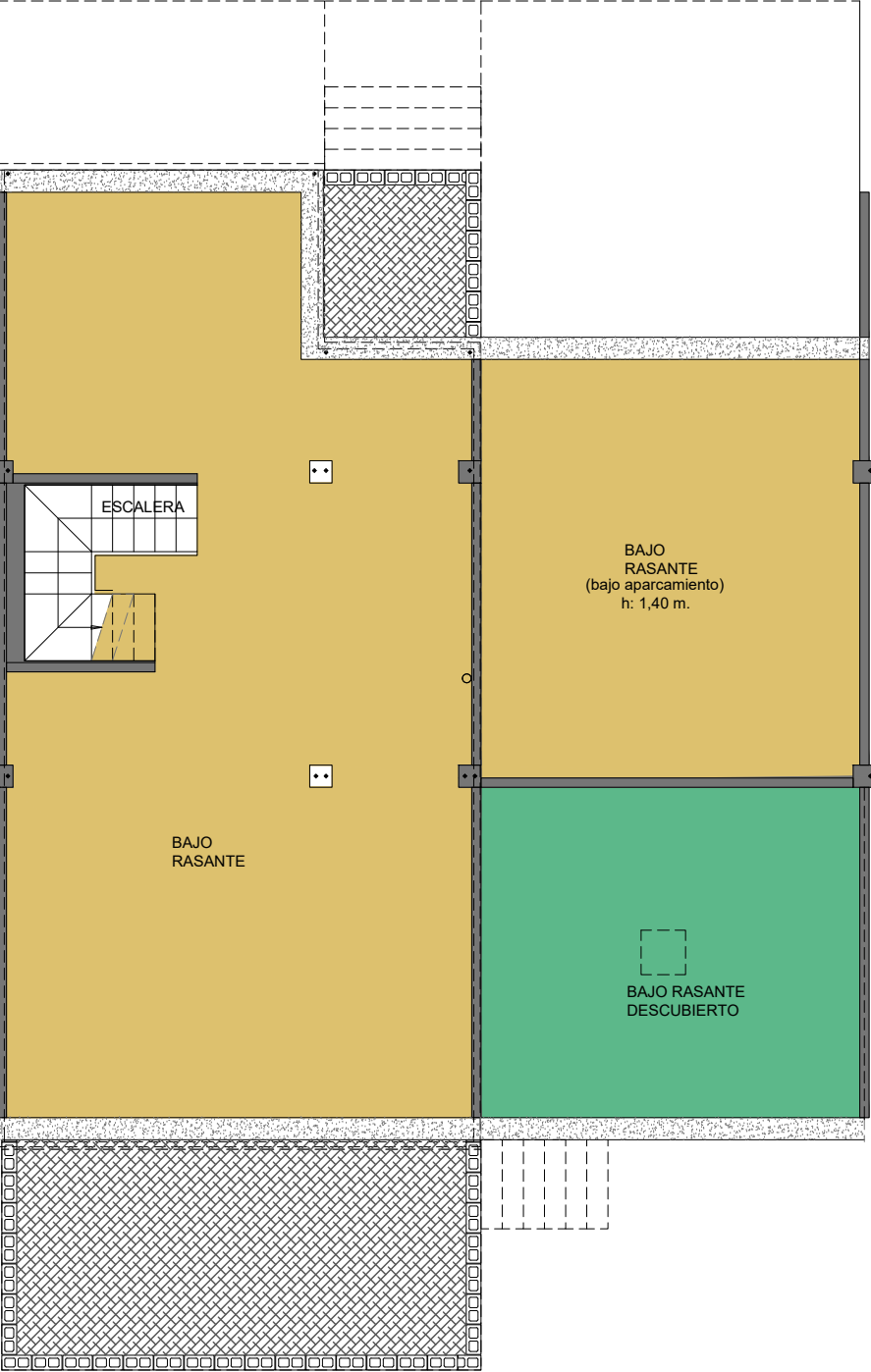
BAJO RASANTE
