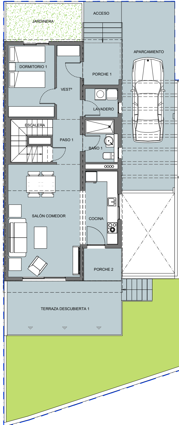
PLANTA BAJA
