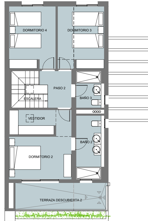
PLANTA PRIMERA
