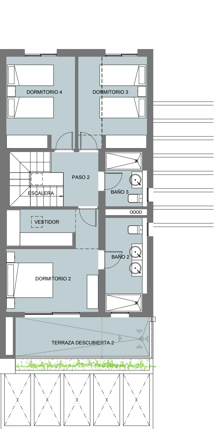
PLANTA PRIMERA
