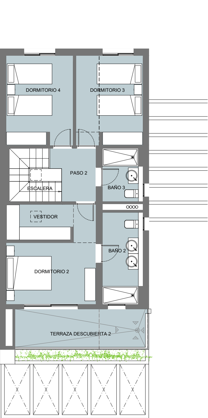
PLANTA PRIMERA
